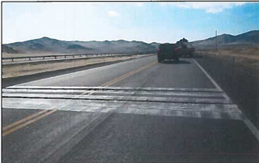
Fotografía 2: Bandas de fresado en operación
